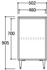
● 開き扉部共通側面図 (50AL/AR・80AD・120AD)
