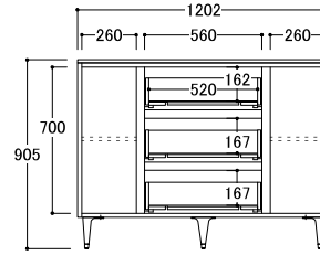
● 共通背板部分詳細図 (開き扉部)
