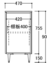
● 開き扉部共通側面図 (50AL/AR・80AD・120AD)
