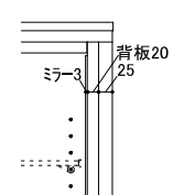
● 共通背板部分詳細図
