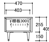
● フラップ扉部共通側面図
