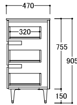
● 引出し部共通側面図 (80AD・120AD)
