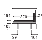
【引き出し部 共通側面図】
