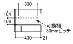
【フラップ扉部 共通側面図】
