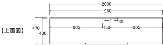
FU-U/FG-G/FD-D200LB ● 外寸 W2000×D470×H383mm
