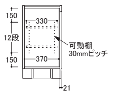
【開き戸部 共通側面図】
