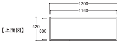
FU-U/FG-G/FD-D120AD ● 外寸 W1200×D420×H783mm
