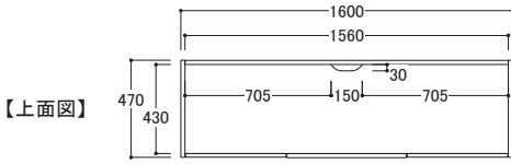
FU-U/FG-G/FD-D160LB ● 外寸 W1600×D470×H383mm
