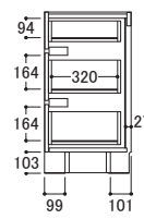
【引き出し部 共通側面図】
