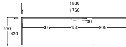
FU-U/FG-G/FD-D180LB ● 外寸 W1800×D470×H383mm
