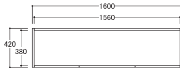
FU-U/FG-G/FD-D160AD ● 外寸 W1600×D420×H783mm
