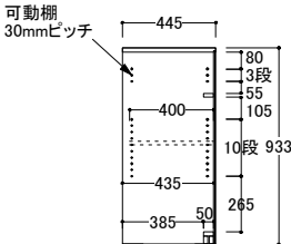
● 共通側面図
