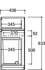
● 共通側面図
