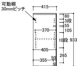
● 共通側面図
