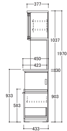
● 側面図
