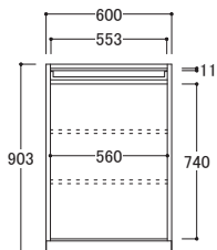
IK/IU-□60CK ● 外寸 W600×D483×H903mm 取手含むD505mm)
