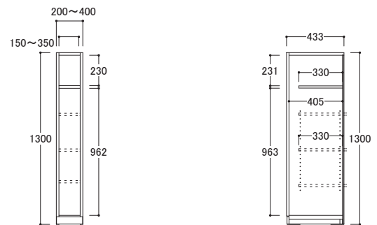
IK/IU-□SBCL2/□SBCR2 ● 外寸 W200~400xD433xH1300mm ● 共通側面図
