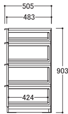
● 共通側面図
