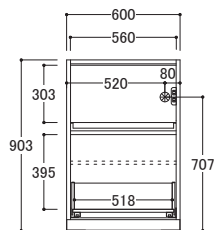
IK/IU-□60G ● 外寸 W600×D483×H903mm 取手含むD505mm)
