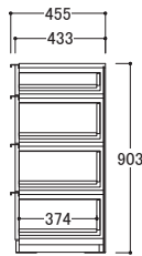
● 共通側面図
