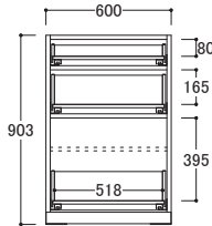
IK/IU-□60D2 ● 外寸 W600×D433×H903mm 取手含むD455mm)
