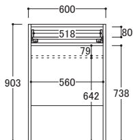
IK/IU-□60B2 ● 外寸 W600×D433×H903mm 取手含むD455mm)
