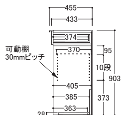
● 共通側面図
