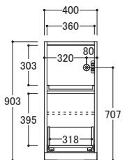
IK/IU-□40G ● 外寸 W400×D483×H903mm 取手含むD505mm)
