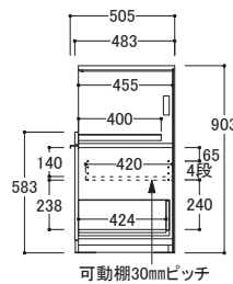
● 共通側面図
