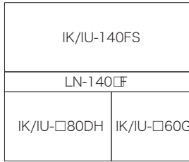
● 外寸 W1402×D500×H1970mm
