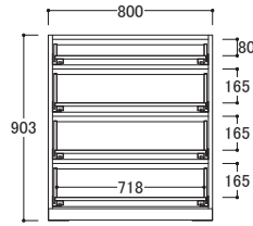
IK/IU-□80DH2 ● 外寸 W800×D433×H903mm 取手含むD455mm)
