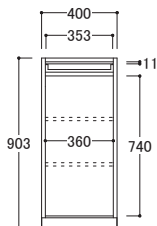
IK/IU-□40CKL/40CKR ● 外寸 W400×D483×H903mm 取手含むD505mm)
