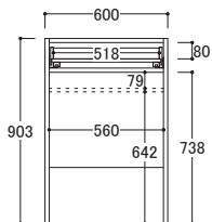
IK/IU-□60B ● 外寸 W600×D483×H903mm 取手含むD505mm)
