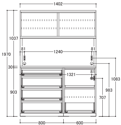
● 外寸 W1402×D450×H1970mm
