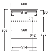
IK/IU-□60BC ● 外寸 W600×D483×H903mm 取手含むD505mm)
