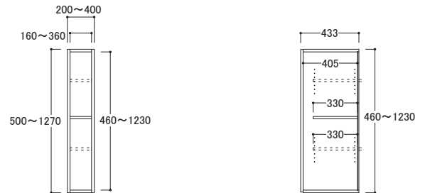
IK/IU-□SBUL2/□SBUR2 ● 外寸 W200~400xD433xH500~1270mm ● 共通側面図
