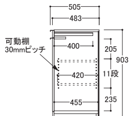
● 共通側面図
