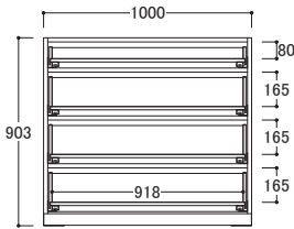
IK/IU-□100DH2 ● 外寸 W1000×D433×H903mm 取手含むD455mm)
