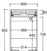
IK/IU-□60BC2 ● 外寸 W600×D433×H903mm 取手含むD455mm)
