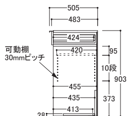
● 共通側面図
