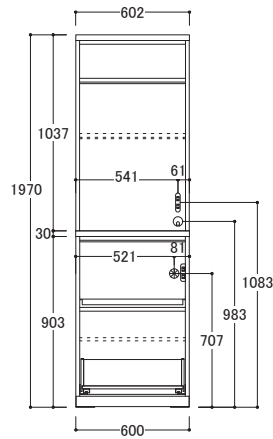
● 外寸 W602×D500×H1970mm
