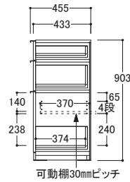
● 共通側面図
