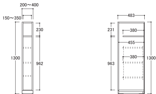
IK/IU-□SBCL/□SBCR ● 外寸 W200~400xD483xH1300mm ● 共通側面図
