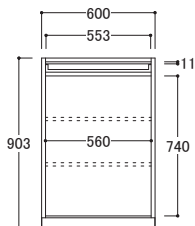
IK/IU-□60CK2 ● 外寸 W600×D433×H903mm 取手含むD455mm)
