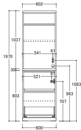
● 外寸 W602×D450×H1970mm
