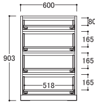
IK/IU-□60DH ● 外寸 W600×D483×H903mm 取手含むD505mm)
