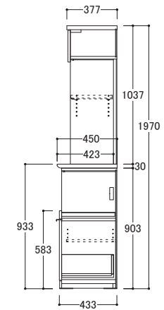
● 側面図
