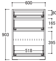
IK/IU-□60D ● 外寸 W600×D483×H903mm 取手含むD505mm)
