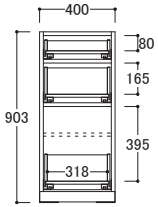
IK/IU-□40D ● 外寸 W400×D483×H903mm 取手含むD505mm)
