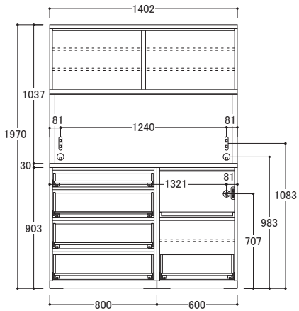
● 外寸 W1402×D500×H1970mm
