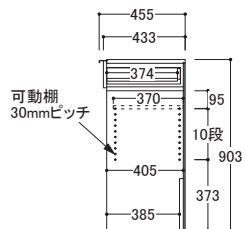
● 共通側面図
