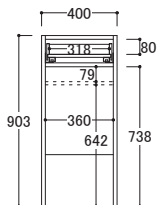
IK/IU-□40B ● 外寸 W400×D483×H903mm 取手含むD505mm)
