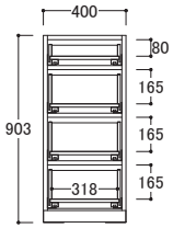
IK/IU-□40DH ● 外寸 W400×D483×H903mm 取手含むD505mm)
