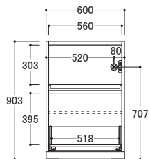
IK/IU-□60G2 ● 外寸 W600×D433×H903mm 取手含むD455mm)
