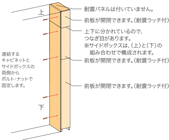
[サイドボックス上下(右)を設置した図]
