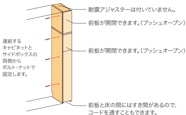
【サイドボックス上下(右)を設置した図】
