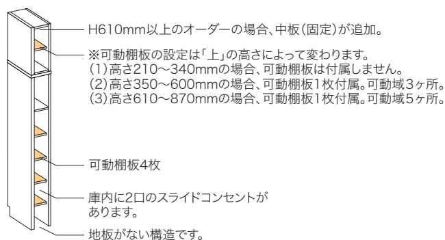
[サイドボックス上下(右)の扉をはずした図]
