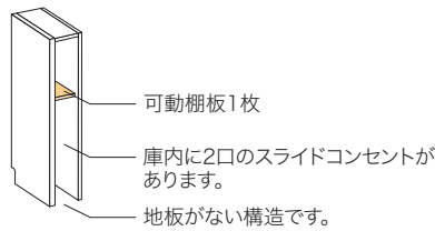
[サイドボックス(右)の扉をはずした図]
